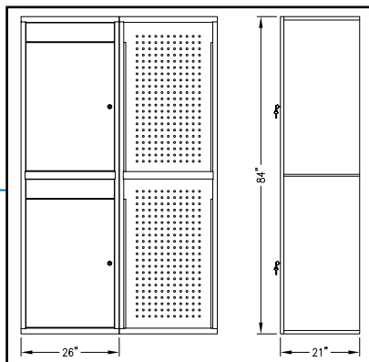
Soiled Garment Disposal Double Tier: 26" x 21" x 84"
